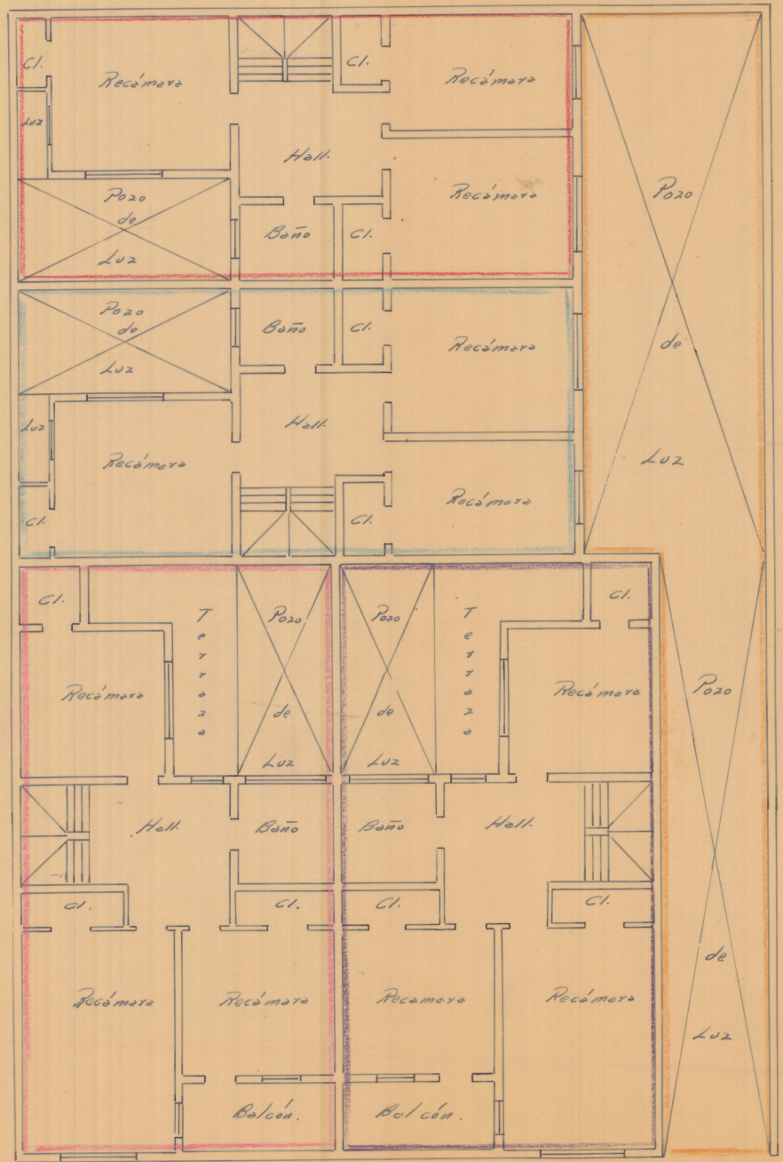
Planta Alta.
