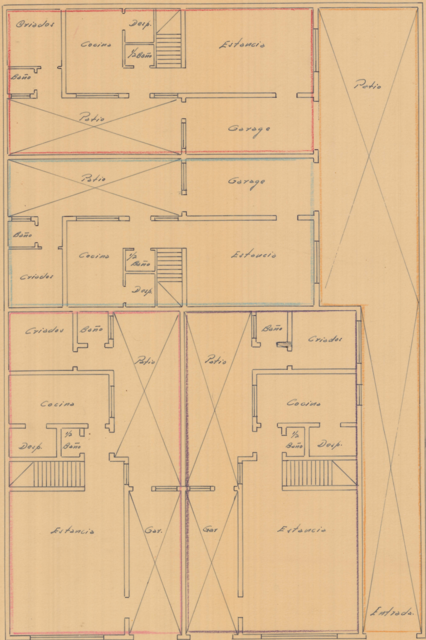
Planta Baja.
